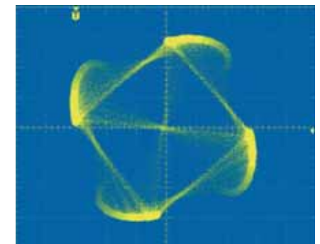
Замирание сигнала 16QAM в канале Рэлея
