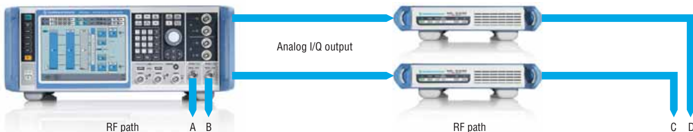
Измерительная установка для 4x4 MIMO, состоящая из двухканального генератора R & S®SMW200A и двух модулей генерации сигналов R & S®SGS100A, управляемых с генератора R & S®SMW200A. Модули обеспечивают ВЧ-тракты 3 и 4. Генератор R & S®SMW200A полностью обеспечивает систему модулирующим сигналом и замираниями.
