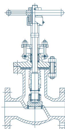
Арматура с сильфонным уплотнением из литой стали
