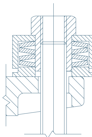
Динамически нагруженный фланец сальника
