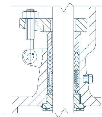
Смазочное кольцо на задвижках и клапанах
