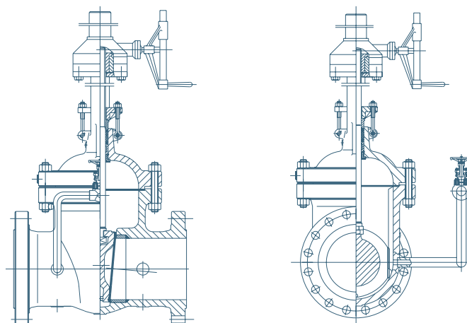
Специальное разгрузочное приспособление
