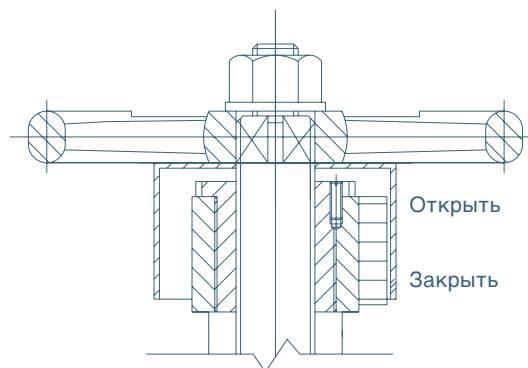
Индикатор положения на клапанах
