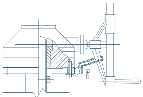
Блокирующее устройство на коробке редуктора
