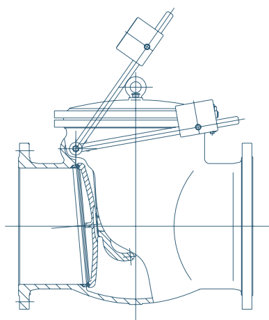
Обратные клапаны с грузовым демпфером
