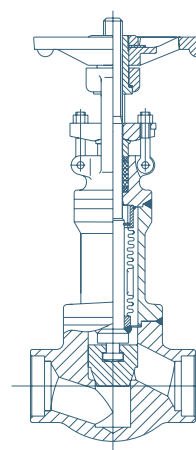
Арматура с сильфонным уплотнением из ковanej стали
