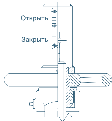
Индикатор положения на задвижках
