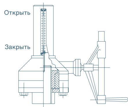
Индикатор положения на коробке редуктора
