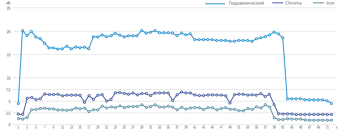
СРАВНЕНИЕ ЭНЕРГОПОТРЕБЛЕНИЯ ГИДРАВЛИЧЕСКИМИ И ЭЛЕКТРИЧЕСКИМИ ПРОБИВНЫМИ СТАНКАМИ
