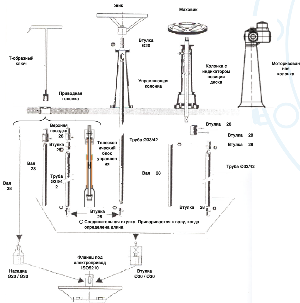
Рисунок 1 Ручной привод
