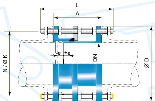
Тип JP DN150-600 Максимально возможное смещение = 2 \times e = 60 - 100 мм
