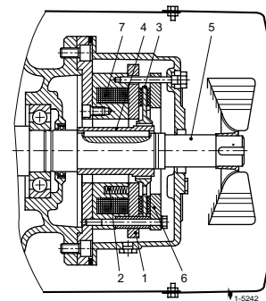
Конструкция тормоза
