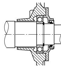
Подшипники с полевой стороны
