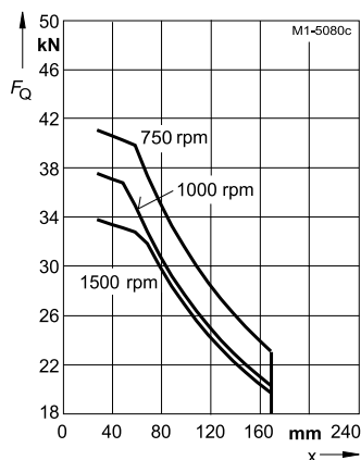
Типоразмер 315, 1LA8 – Монтажное исполнение IM B 3
