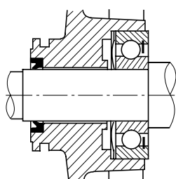
Рис. 1 Подшипники со стороны рабочего вала
