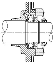
Подшипники с полевой стороны
