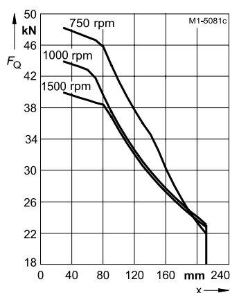
Типоразмер 355, 1LA8 – Монтажное исполнение IM B 3
