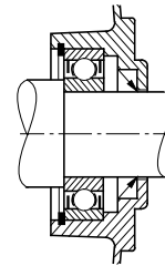
Подшипники с полевой стороны
