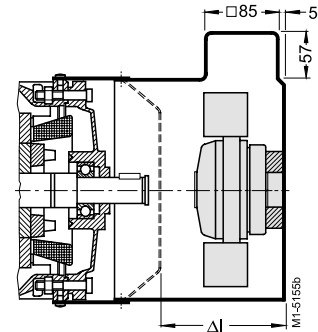
Вентилятор принудительного охлаждения, Код Заказа G17
