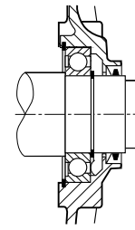
Подшипники с полевой стороны
