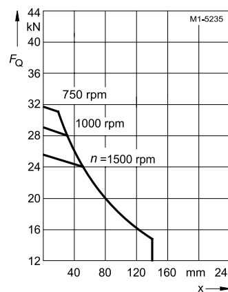
Типоразмер 280, 4- to 8-pole, 1LG4/1LG6
