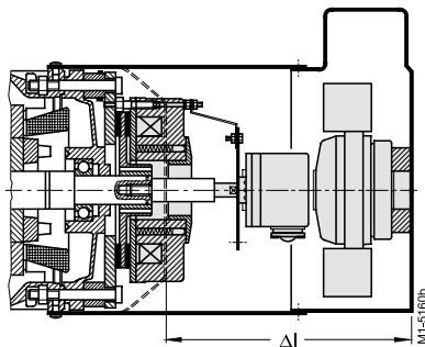
Тормоз, импульсный датчик скорости вентилятор принудительного охлаждения, Код заказа H64, H99
