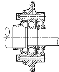
Подшипники с полевой стороны
