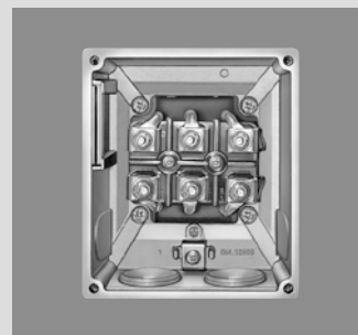
Тип gk330 для 1LA5, 1LG4
