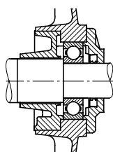
Подшипники с полевой стороны
