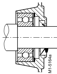
Подшипники с полевой стороны
