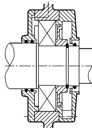
Подшипники с полевой стороны
