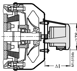
Импульсный датчик скорости, Код заказа H57, H58, H70, H72, H73
