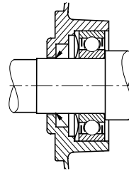
Рис. 4 Подшипники со стороны рабочего вала
