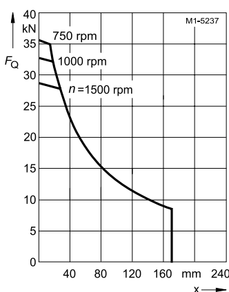
Типоразмер 315S/M, 4- to 8-pole, 1MA6
