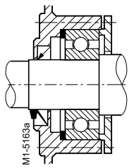
Рис. 3 Подшипники со стороны рабочего вала
