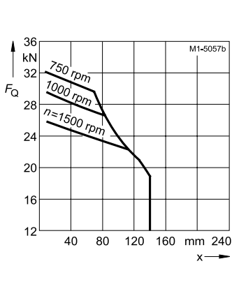
Типоразмер 280, 4- to 8-pole, 1MA6
