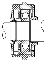
Рис. 5 Подшипники со стороны рабочего вала
