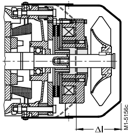
Тормоз и импульсный датчик скорости, Код заказа H62, H98
