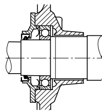
Рис. 4 Подшипники со стороны рабочего вала
