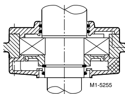
Рис. 7 Подшипники со стороны рабочего вала
