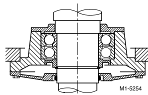
Подшипники с полевой стороны
