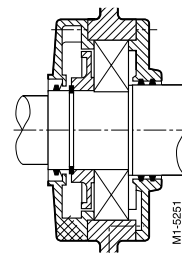
Рис. 6 Подшипники со стороны рабочего вала
