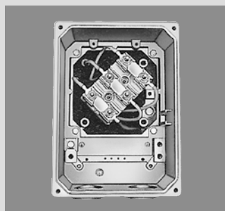
Тип gk430, gt431
