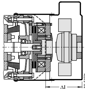
Тормоз и вентилятор принудительного охлаждения, Код заказа H63
