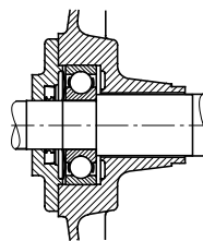
Рис. 2 Подшипники со стороны рабочего вала
