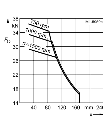
Типоразмер 315L, 4- to 8-pole, 1MA6
