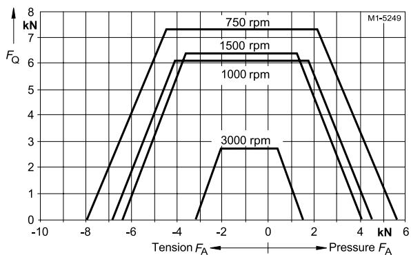
Типоразмер 400, 1LA8 – Монтажное исполнение IM B3
