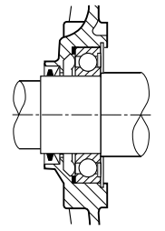
Рис. 4 Подшипники со стороны рабочего вала
