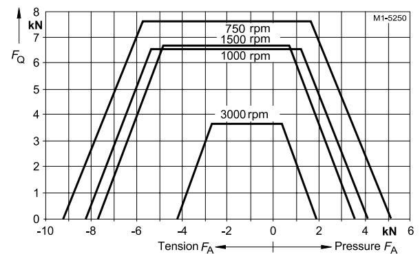
Типоразмер 450, 1LA8 – Монтажное исполнение IM B3
