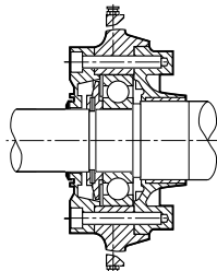
Рис. 6 Подшипники со стороны рабочего вала
