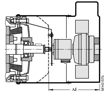
Импульсный датчик скорости и вентилятор принудительного охлаждения, Код заказа H61, H97
