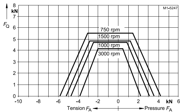
Типоразмер 315, 1LA8 – Монтажное исполнение IM B3
