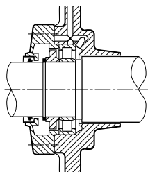
Рис. 5 Подшипники со стороны рабочего вала
