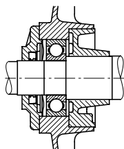
Рис. 3 Подшипники со стороны рабочего вала
