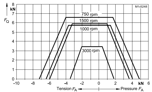
Типоразмер 355, 1LA8 – Монтажное исполнение IM B3
