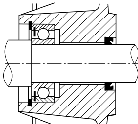
Подшипники с полевой стороны
